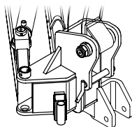
Selbsteinsteuerndem Gelenk
