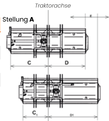
Stellung b
