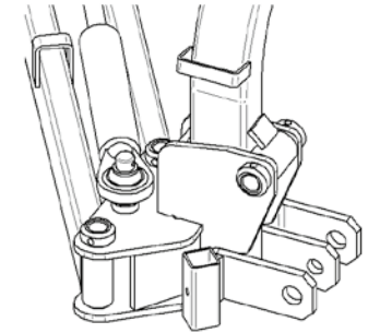
Selbstfeinsteuerndes Gelenk
